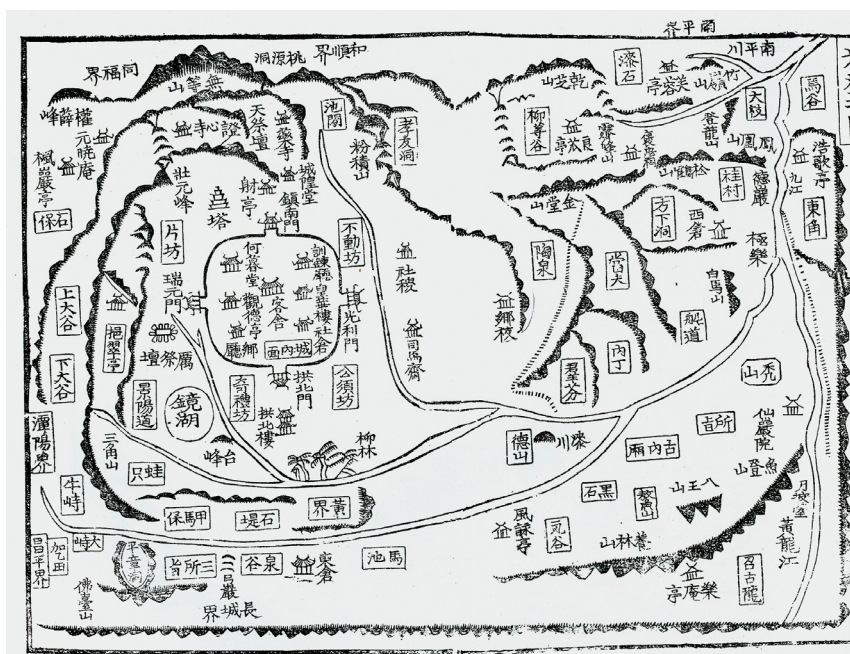
광주의 옛 지도(1879년)
